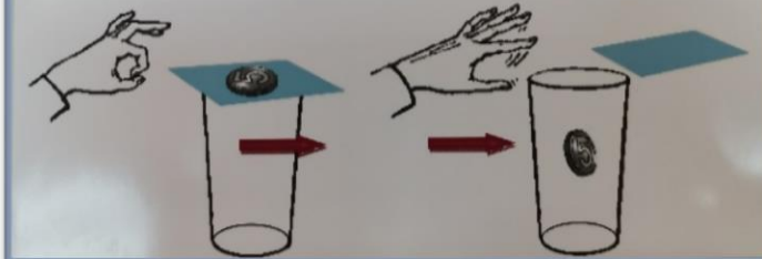
Опыт №4 «Монетка-попрыгунья»
